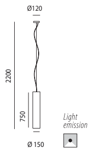
Sospensione - Pendant lamp
