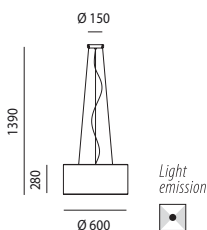
Sospensione - Pendant lamp
