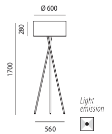
Lampada da terra - Floor lamp
