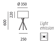
Lampada da tavolo - Table lamp
