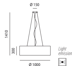
Sospensione - Pendant lamp
