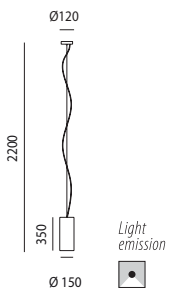
Sospensione - Pendant lamp
